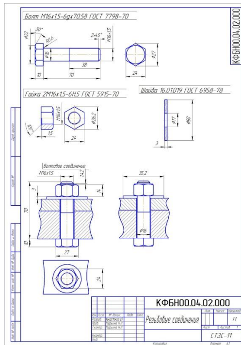
Пример выполнения резьбовых соединений
