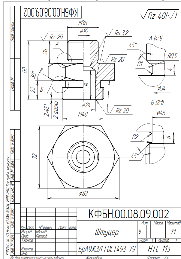
Пример выполнения рабочего чертежа детали второй сложности
